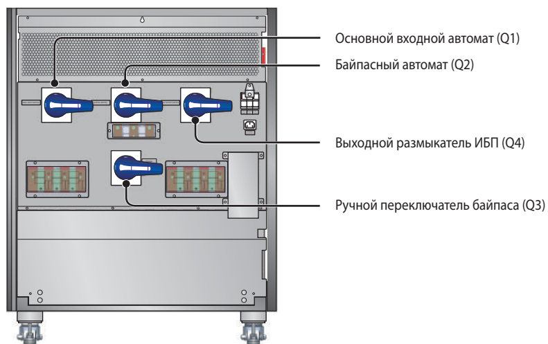
Рис. 2-н. Входные и выходные выключатели
