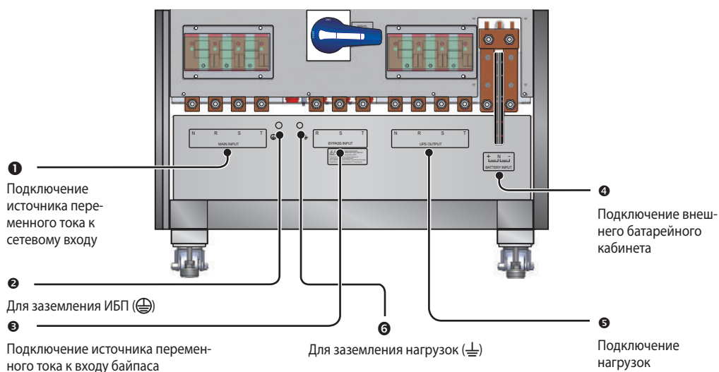
Рис. 2-т. Выводы ИБП
