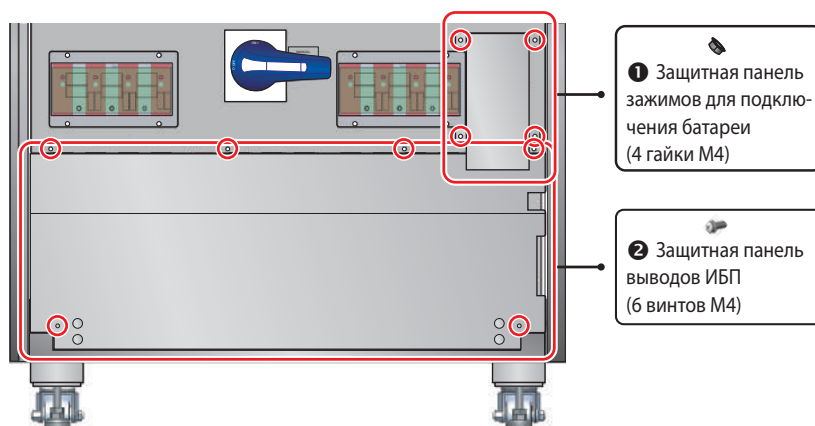
Рис. 2-1. Расположение защитных панелей
