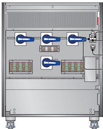
Рис. 2-г: Держатели предохранителей вспомогательного питания, выхода переменного тока и вентилятора
