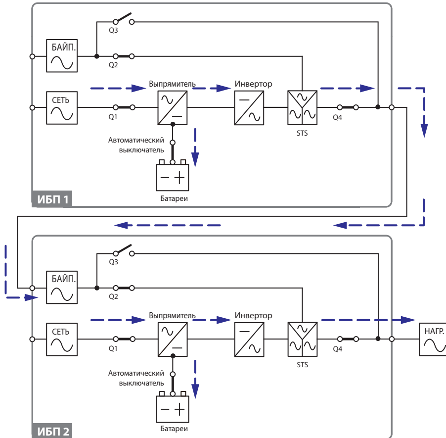
Рис. 3-ж. Передача электроэнергии через параллельные ИБП в системе с последовательным резервированием
