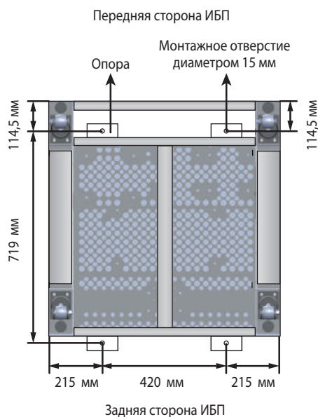
Рис. 2-с. Вид снизу и расположение крепежных отверстий
