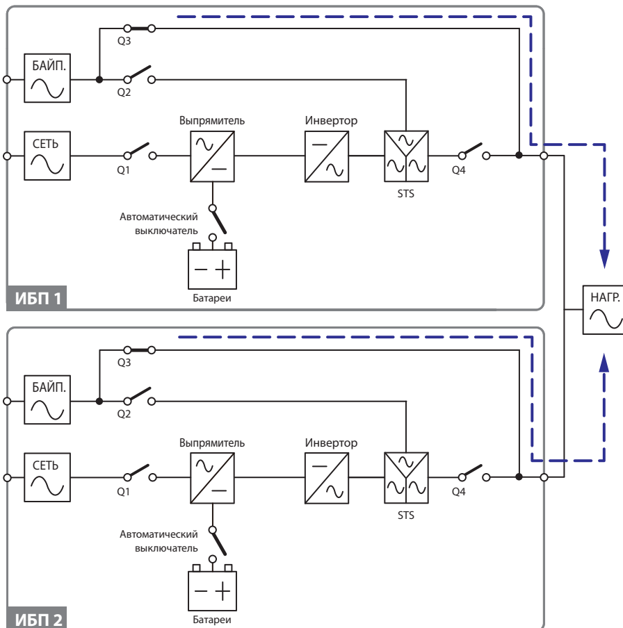
Рис. 3-і. Передача электроэнергии через параллельные ИБП в режиме ручного байпаса
