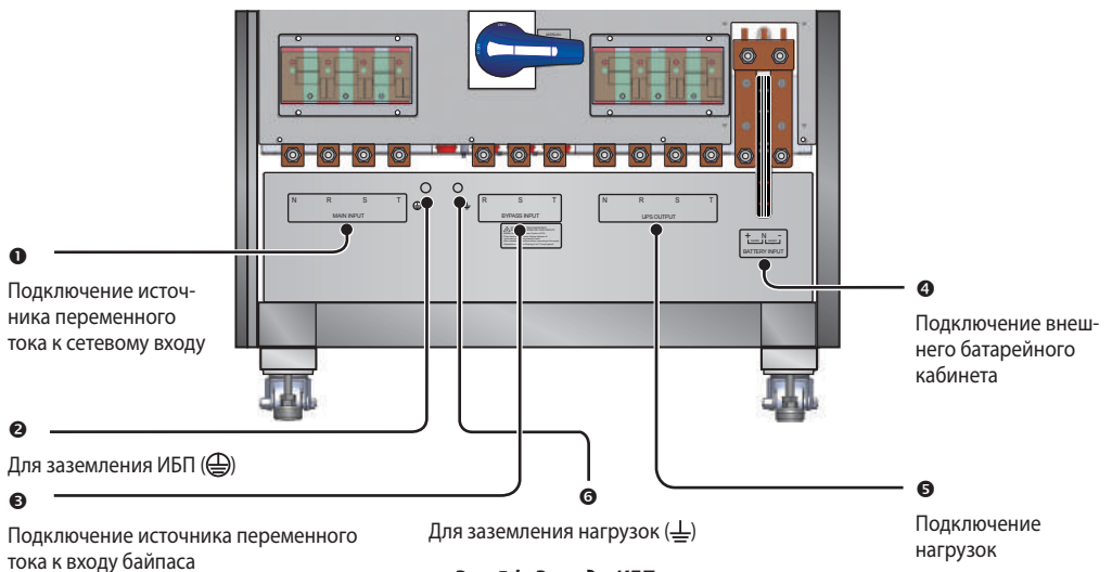
Рис. 5-к. Выводы ИБП
