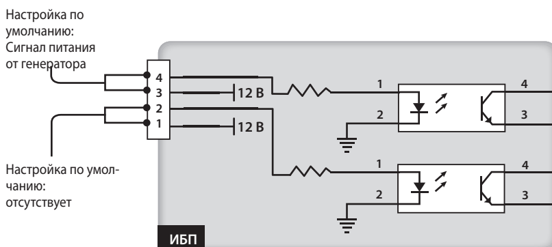
Рис. 4-д. Входы с сухими контактами (два комплекта)
