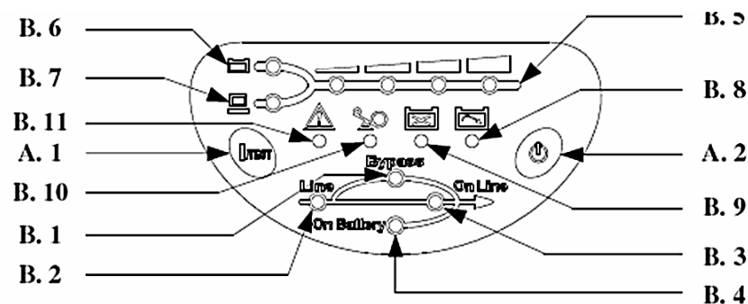
Рис. 2-2 Панель управления
