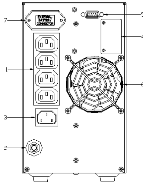
Рис. 2-3 ИБП мощностью 1 кВА
