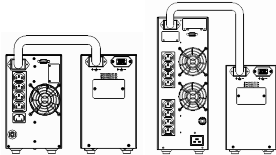
Рис. 3-2.1 ИБП мощностью 1 кВА
