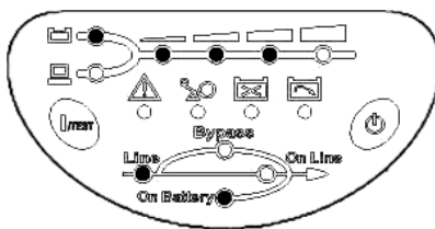
Рис. 4-3 Панель управления в режиме самопроверки
