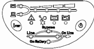
Рис. 4-8 Индикация короткого замыкания на выходе ИБП
