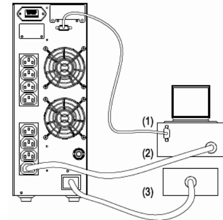
Рис. 3-3.2 Подключение ИБП мощностью 2 кВА и 3 кВА
