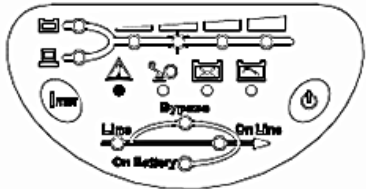
рис. 4-9 «Недостаточное выходное напряжение»
