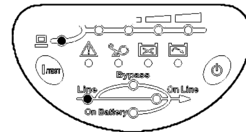
Рис. 3-1 Панель управления в дежурном режиме
