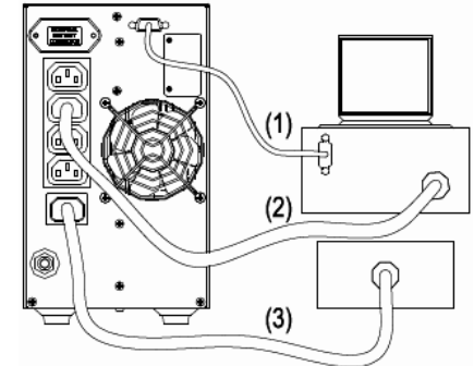
Рис. 3-3.1 Подключение ИБП мощностью 1 кВА
