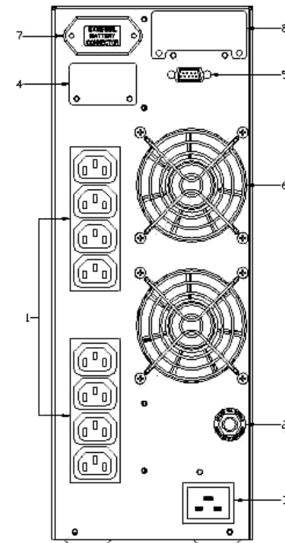
Рис. 2-4 ИБП мощностью 2 кВА и 3 кВА
